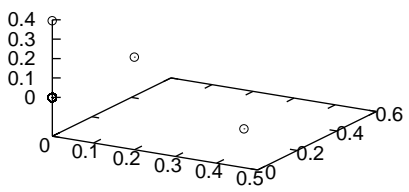
AP214 - TFIDF
