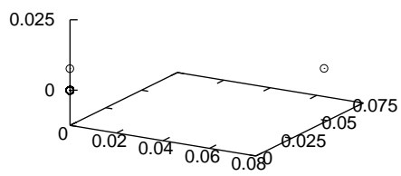
AP203 - TFIDF
