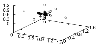
AP214 - FastMap
