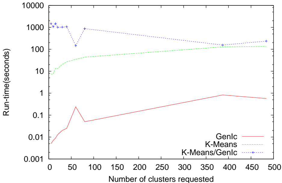
K-Means vs Genlc - STEP ap203 (n=484)
