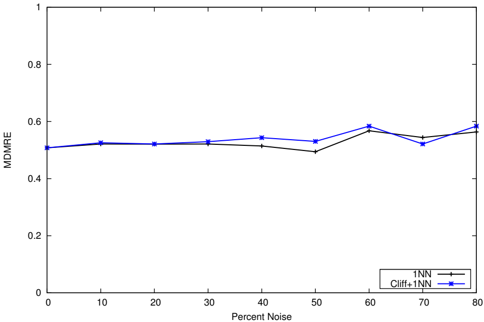
MDMRE for isbsg
