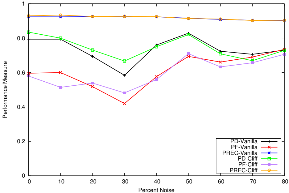
cm1 - false
