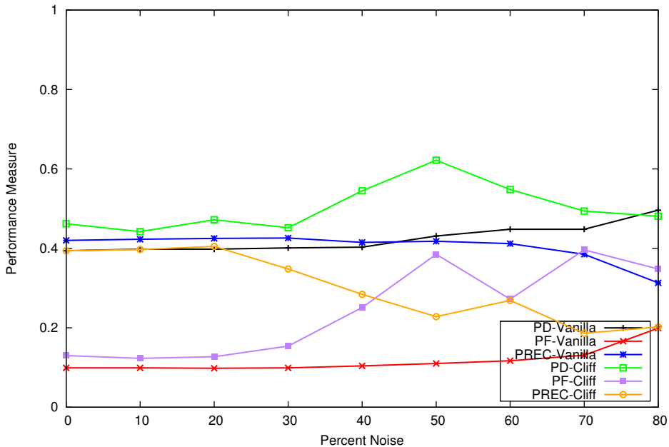
kc1 - true
