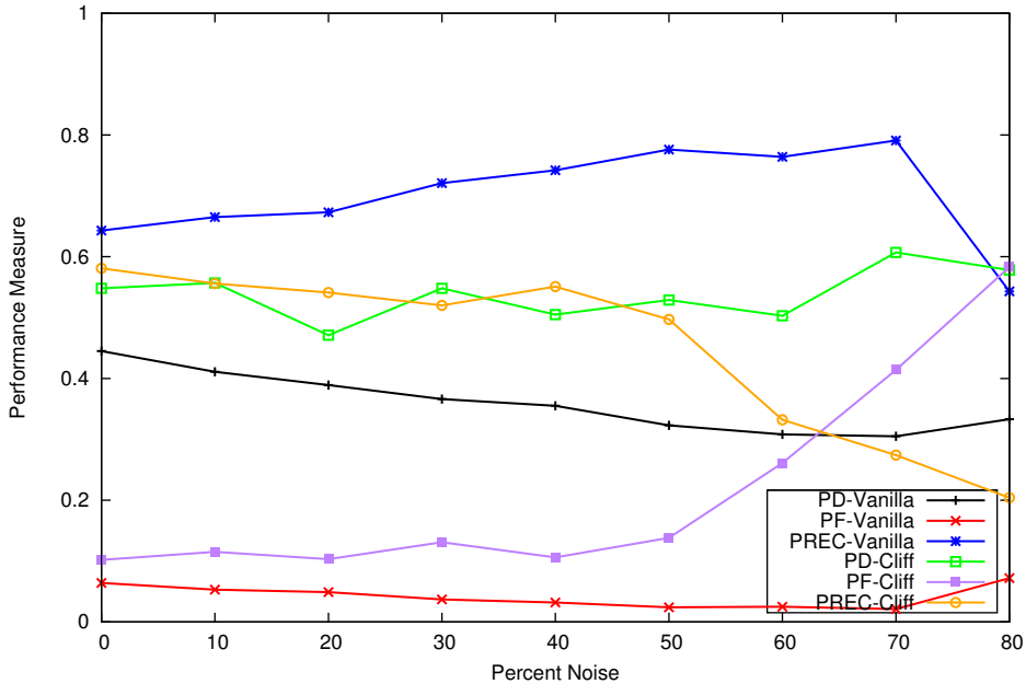
kc2 - true
